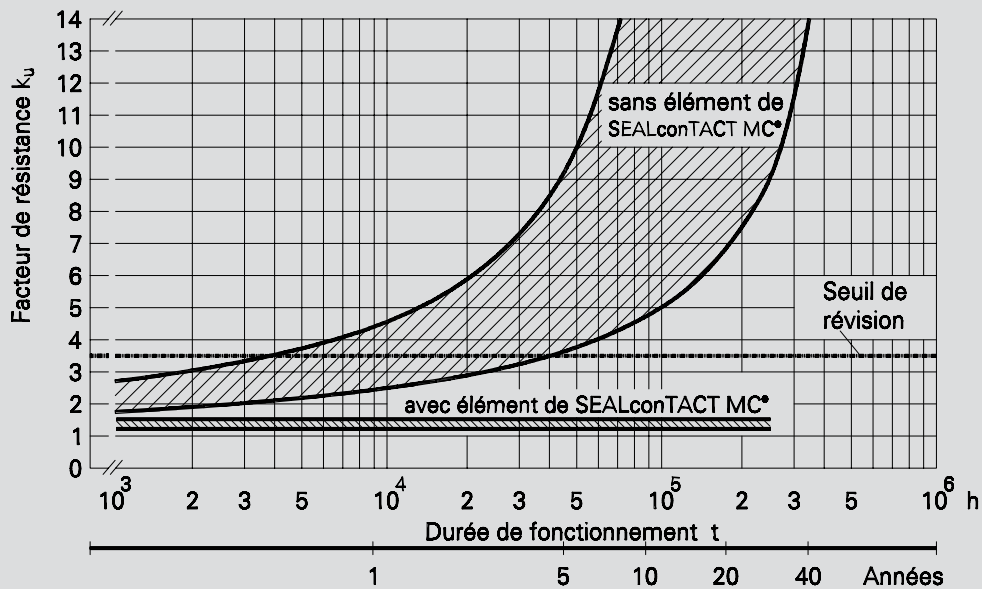
Figure 5 Facteur de résistance à long terme k_u(t)
